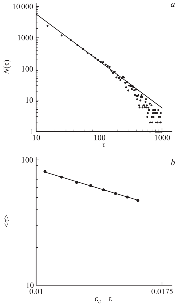
Рис. 1. Распределение длительности ламинарных фаз при \varepsilon = 0.1525 (а) и зависимость средней длительности ламинарных фаз \langle \tau \rangle от параметра надкритичности (\varepsilon_c - \varepsilon) , \varepsilon_c = 0.1625 логистических отображений (3), находящихся вблизи границы индуцированной шумом синхронизации, и соответствующие аппроксимации степенными законами (1) (а) и (2) (б). Данные, полученные путем численного моделирования, показаны точками, теоретические зависимости — сплошными линиями.
