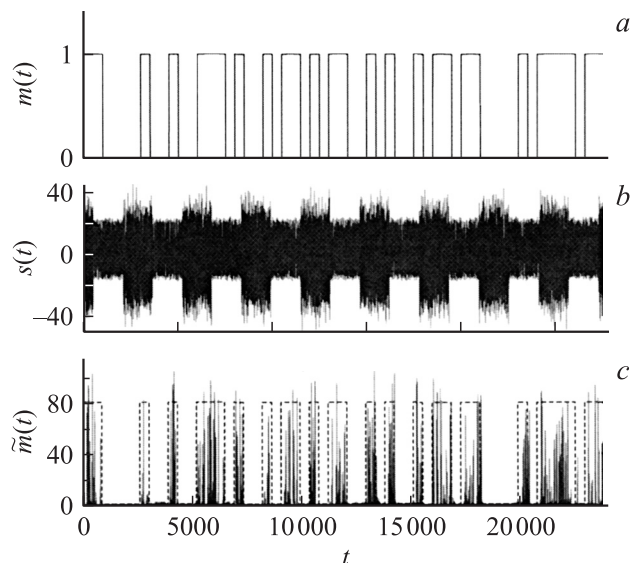
Рис. 5. Иллюстрация работоспособности метода скрытой передачи информации на основе режима обобщенной синхронизации в присутствии шума в случае, если характеристики генератора шума модулируются последовательностью бинарных битов: информационный сигнал m(t) , представленный последовательностью бинарных битов 0/1 (a), сигнал s(t) , передаваемый по каналу связи (b), восстановленный сигнал \hat{m}(t) (c), сплошная линия. На рисунке представлен также детектированный информационный сигнал (пунктир).
