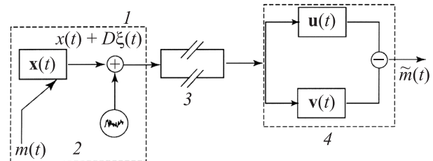
Рис. 1. Схема для реализации способа скрытой передачи информации на основе режима обобщенной хаотической синхронизации в присутствии шума (1 — передающее устройство, 2 — генератор шума, 3 — канал связи, 4 — принимающее устройство).
