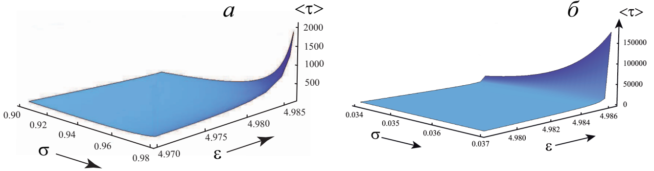
Рис. 3: (а) Зависимость средней длительности участков ламинарного поведения от двух параметров надкритичности ( \epsilon и \sigma ) для системы, демонстрирующей одновременное сосуществование двух типов перемежаемости кольца; (б) Зависимость средней длительности ламинарного поведения от двух параметров надкритичности ( \epsilon и \sigma ) для системы, демонстрирующей одновременно два типа перемежающегося поведения: тип “кольцо” и тип игольного ушка
