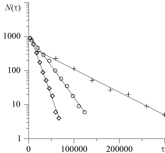
Рисунок 5 — Распределения длительности ламинарных фаз однонаправленно связанных диодов Пирса от времени. Точки, соответствующие значению параметра связи \varepsilon = 0.0075 , показаны символами “◇”, значению \varepsilon = 0.008 — символами “○”, значению \varepsilon = 0.0085 — символами “+”.
